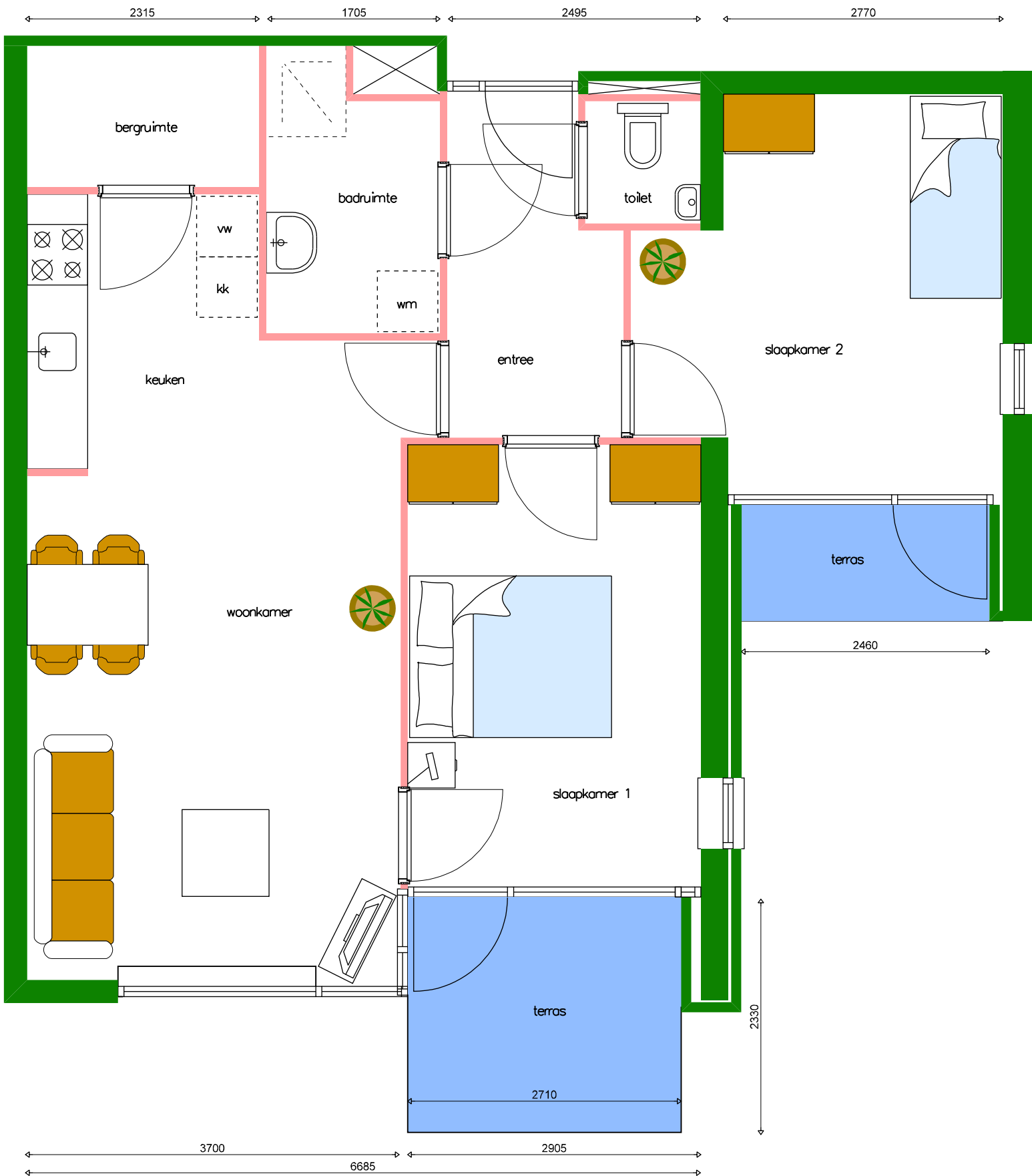
NIEUW VERLAAT - 3 kamerwoning TYPE B1
