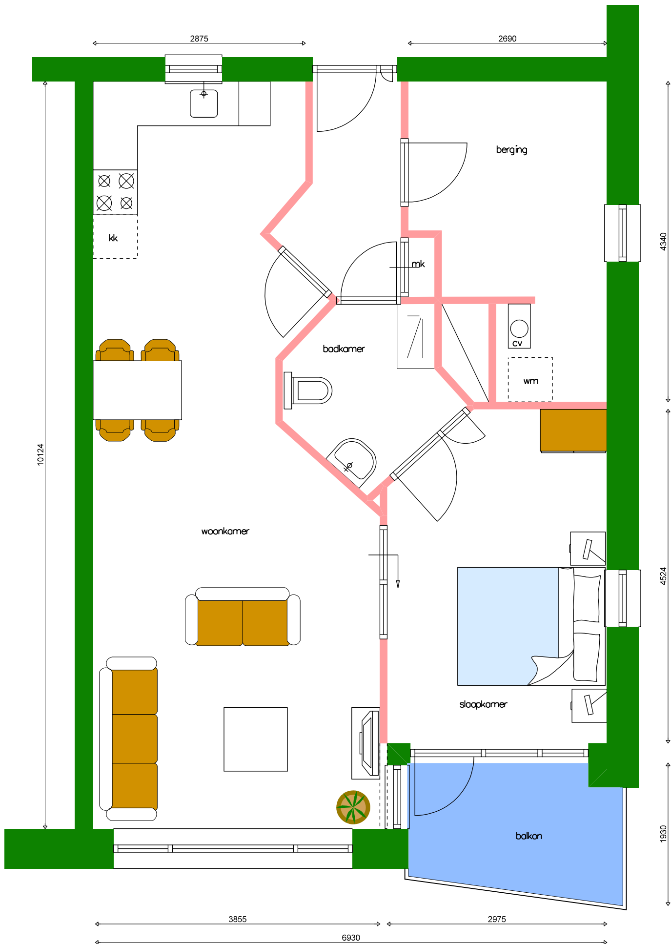
RAVENSWAARD - 2 kamerhoekwoning TYPE CD
